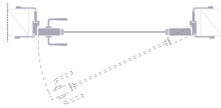
Правое открывание
